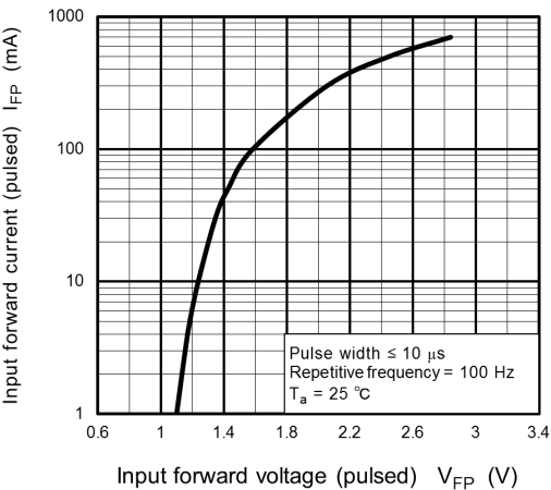
Fig. 11.6 I_{FP} - V_{FP}
