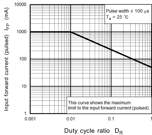
Fig. 11.3 I_{FP} - D_R
