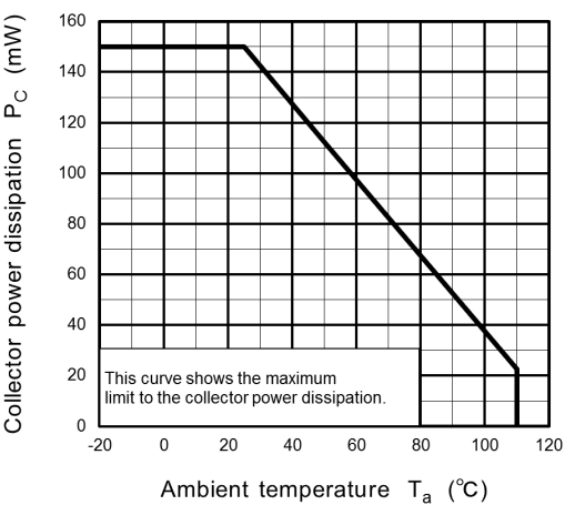
Fig. 11.2 P_C - T_a
